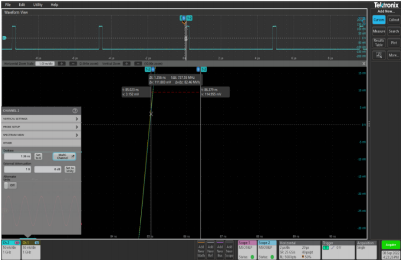
图 14: 在通道垂直徽章标志的“Deskew”（相差校正）设置中输入测得的差量时间，可将校正两个通道之间的相差。
