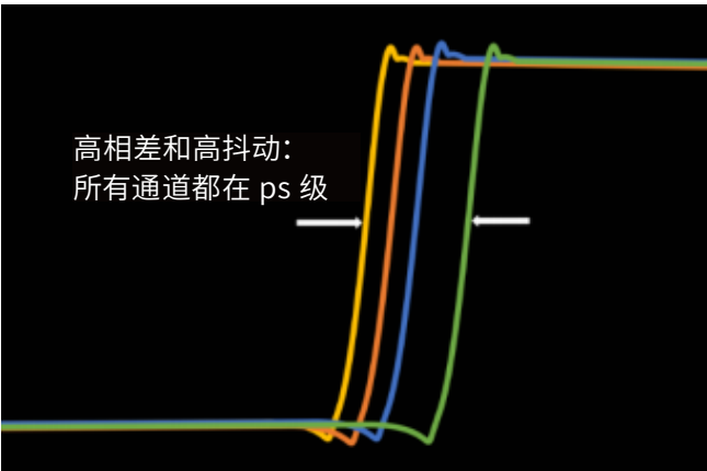
图 1d: 高相差和高抖动 (最差)。
