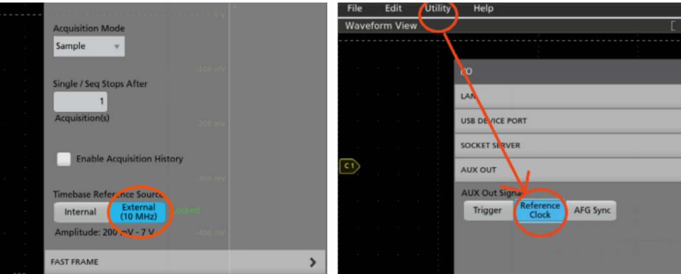
图 6: 4, 5 和 6 系列 MSO 菜单，用于设置参考时钟并锁定时基参考。左侧是接收示波器上参考时钟设置。右侧是发射示波器上的输出参考时钟的设置。
