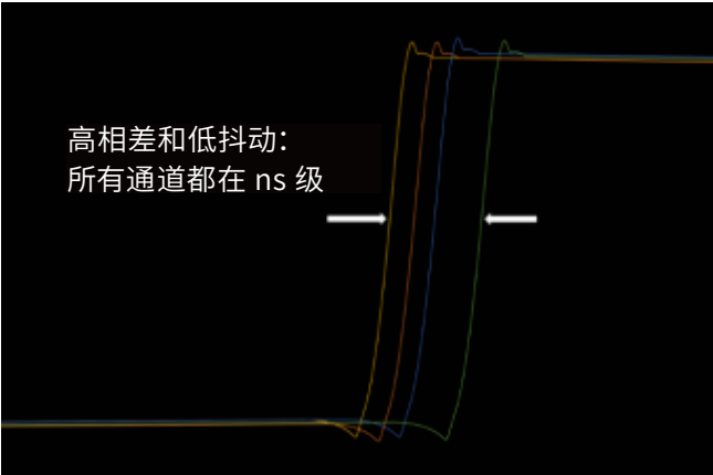
图 1b: 高相差和低抖动。
