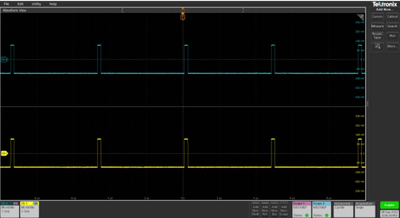
图 11: 相同的信号接入到待校正相差的两个通道。
