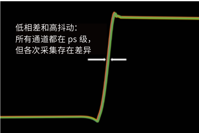
图 1c: 低相差和高抖动。
