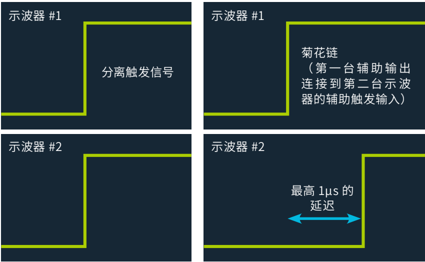
图 2: 不同的触发设置导致不同的相差或延迟。左侧的设置将同一个触发信号使用相位匹配电缆馈送至两台仪器的触发通道。右侧的设置显示了“菊花链”的影响，其中一台示波器的辅助输出馈送至下一台示波器的辅助触发输入通道，导致明显的延迟。
