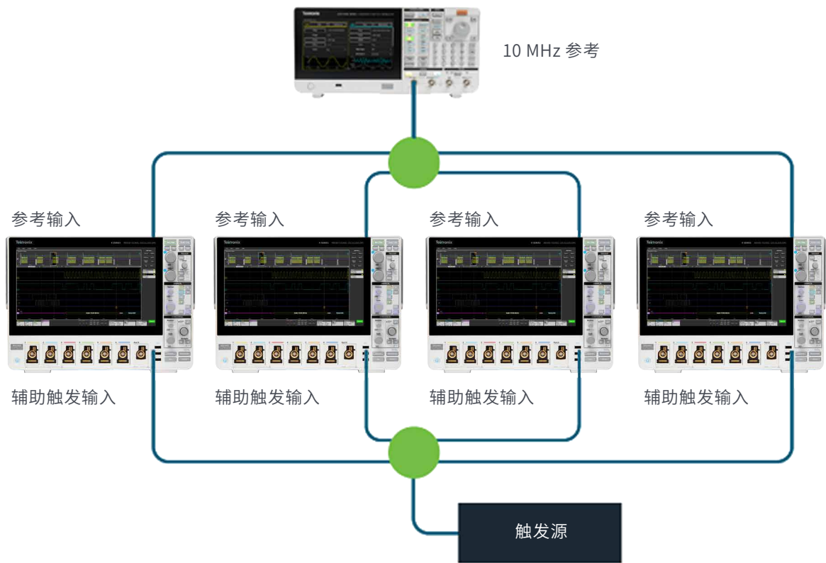
图 3: 该系统中, 辅助触发输入和时基参考均由分离器和匹配的 50Ω 电缆馈送。此设置在不牺牲每台示波器通道的情况下提供了最佳相差结果。使用输入通道代替辅助触发输入将减少测量通道的数量, 但触发抖动会减少大约 200 ps。
