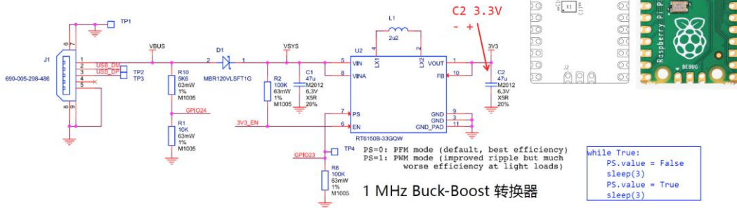
图 1: Raspberry Pi Pico 的供电电路
