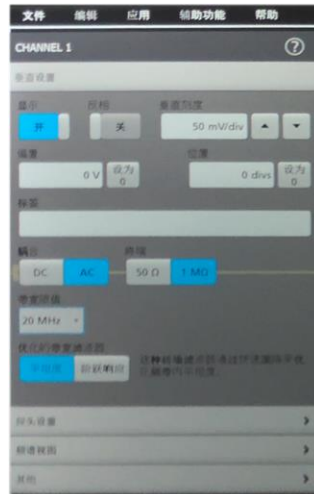
图 2: 示波器垂直通道设置
