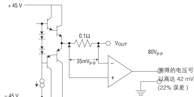
图 6.9. CMRR 为 10,000:1 的差分放大器的共模误差。
