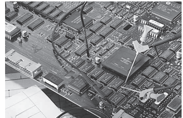
a. 探测 SMT 设备。
