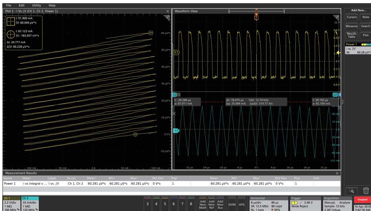
图 5. I 相对于 Jv 关系测量可以进一步了解电感器性能。设计人员可以看到在多个周期中累积的任何 DC 偏置。黄色波形 (CH1) 是经过电感器的电压，蓝色波形 (CH2) 是流经电感器的电流。
