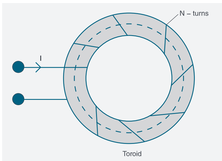
图 2. 基本电感器 - 在封闭的铁磁芯上缠一个线圈。I 安培电流流经 N 圈的线圈。线圈的电感描述了线圈中流动的电流与磁通量之间的关系。
