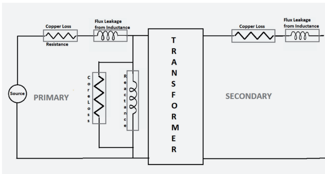
图 10. 变压器损耗可以建模为多个线性单元组合。
