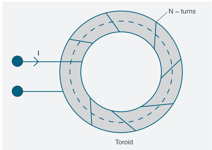
图 2. 基本电感器 - 在封闭的铁磁芯上缠一个线圈。I 安培电流流经 N 圈的线圈。线圈的电感描述了线圈中流动的电流与磁通量之间的关系。
