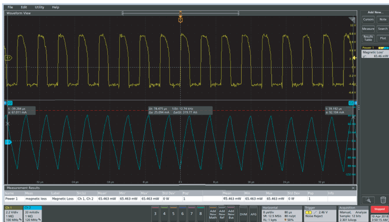
图 11.5—PWR 磁损耗测量给出了总磁损耗，包括磁芯损耗和铜缆损耗。设计人员可以从器件制造商的产品技术资料中找到磁芯损耗，再从总磁损耗中减去磁芯损耗，得到铜缆损耗。
