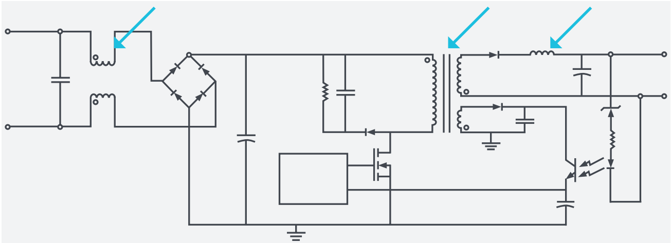
图 1. 电感器和变压器在开关式电源中发挥着关键作用，包括滤波、升压 / 降压、隔离、能量贮存和振荡。
