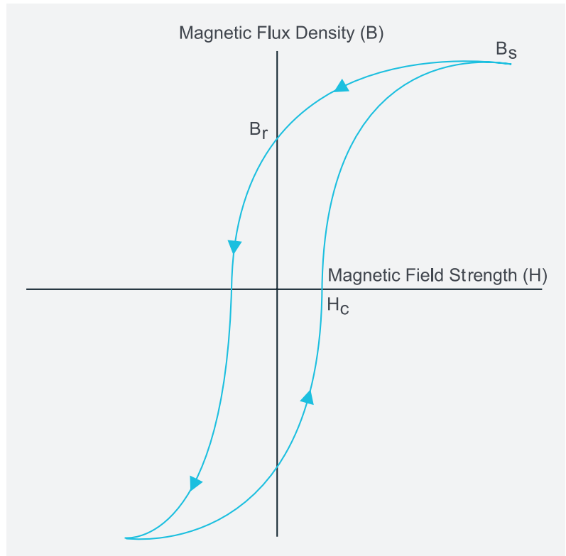
图 6. 典型的 B-H 曲线或“磁滞曲线”。磁芯材料制造商可能会作为技术指标的一部分，提供这样的磁滞曲线。
