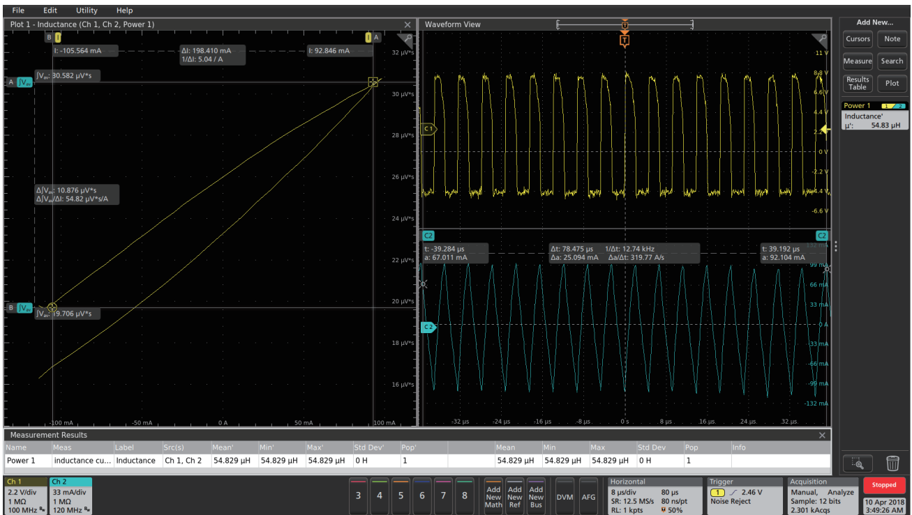
图 4. 电感测量给出了平均电感值，单位为亨利。黄色波形 (CH1) 是经过电感器的电压，蓝色波形 (CH2) 是流经电感器的电流。左图显示了电流 i 相对于 \int v dt 的关系，其斜率就是电感。
