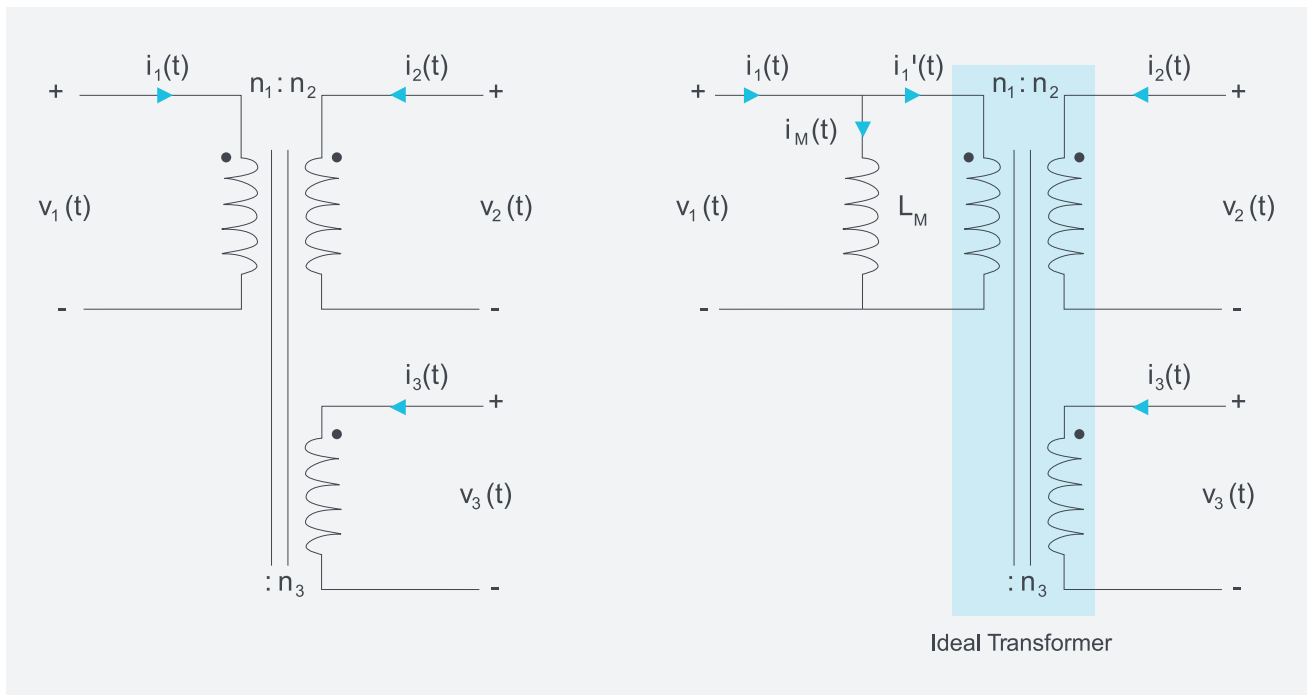
图 9. 变压器示意图 (左) 和等效电路 (右), 显示流经虚数电感器的磁化电流, L_M 与一级线圈并联。LM 建立变压器的磁性特点模型。
