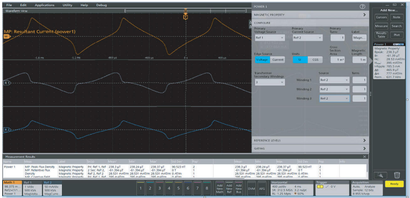
图 8. 多个二级线圈变压器上的磁测量。Ref1 (白色) 波形是经过电感器的电压，Ref 2 (蓝色) 波形是电感器电流。数学波形 (橙色) 是得到的电流波形，是在用户配置测试多个二级线圈时创建的。
