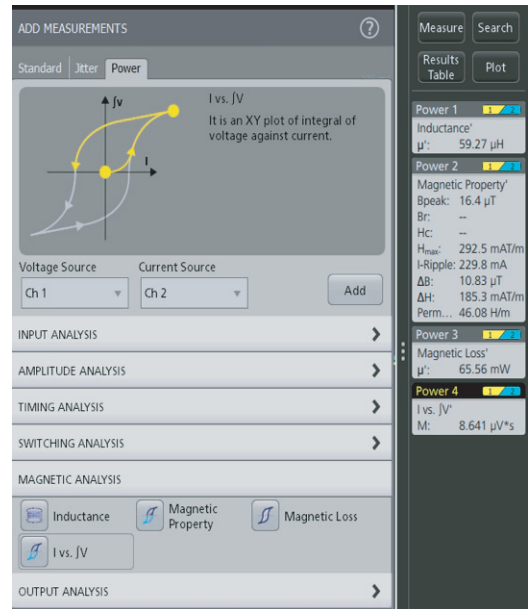
图 3. 指定电压通道和电流通道，设置电感和 i 相对于 \int v 关系测量。
