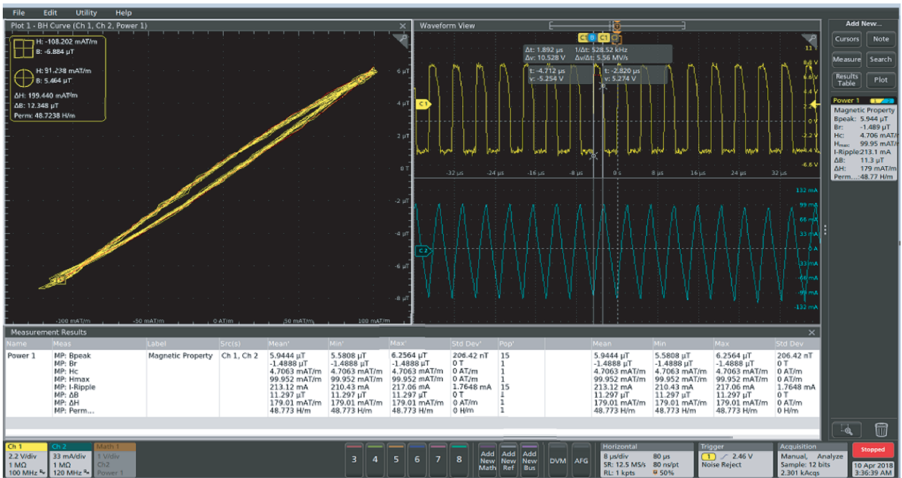
图 7.5–PWR 磁属性测量给出了设计中的磁性器件的磁滞回线，检查磁性器件是否饱和，因为会导致电源不稳定。
