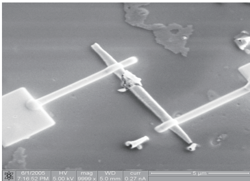
上图为融化断裂的纳米管，由于施加电流过大自热引起断裂
